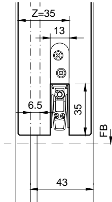
Typ: RDS17-43 48-51mm Türblatt (Zusatzfalz = 15mm)
