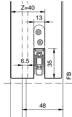
Typ: RDS17-48 58-61mm Türblatt (Zusatzfalz = 20mm)
