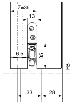
Typ: RDS14-28/33H,F 68-72mm Türblatt (Zusatzfalz = 16mm)
