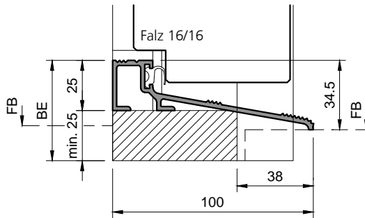
Typ: GS-165 (für Aussentüren, gegenöffnend) Achtung: Rahmendicke fix 90mm!
