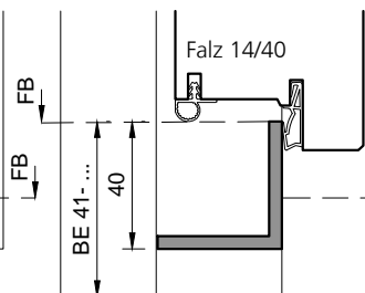
Typ: TT40S (Schwellenwinkel)
