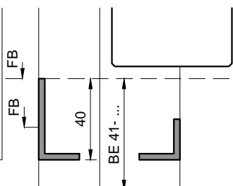
Typ: S (auf FS) (Konterschwelle)
