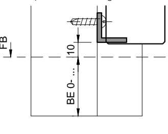
Typ VP (prov. Verbindungsisen)
