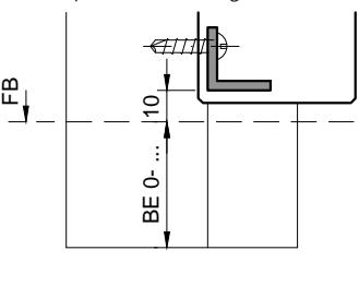
Typ VP (prov. Verbindungsseisen)
