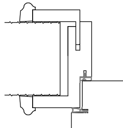
Variante/Beispiel: Zierleiste Typ B
