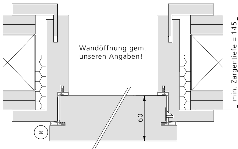
Variante/Beispiel: Zierleiste Typ O
