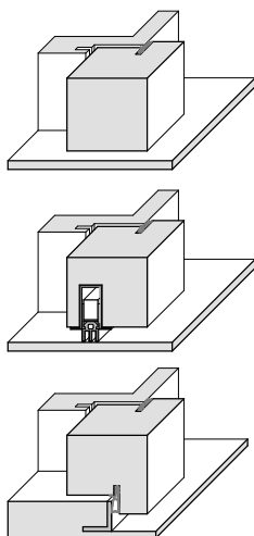
schwellenlos, Bodensenk- dichtung, Winkelschwelle
