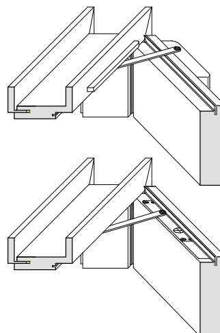
Option: aufgesetzter oder integrierter Türschliesser
