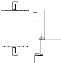
Variante/Beispiel: Zierleiste Typ O
