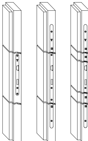
Einsteckschloss, 4-Punkt-, 6-Punkt-Verriegelung
