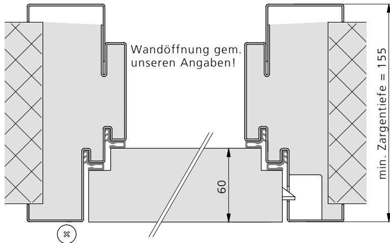
Variante/Beispiel: Stoss in der Leibung
