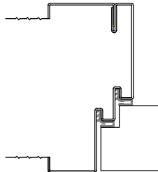
Variante/Beispiel: Stoss im Spiegel
