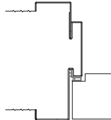
Variante/Beispiel: Zarge mit Einfachfalz
