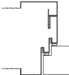
Variante/Beispiel: Stoss in der Leibung
