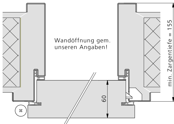
Variante/Beispiel: Spiegelverbreiterung
