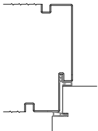
Variante/Beispiel: Schatten-Nut
