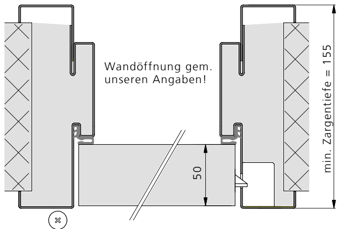
Variante/Beispiel: Stoss in der Leibung
