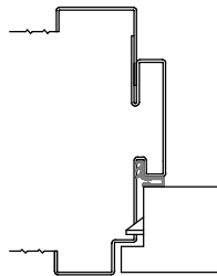
Sicherheitsfalz auf Schloss-Seite
