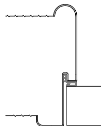
Variante/Beispiel: Rundspiegel
