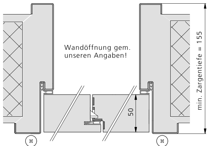
Variante/Beispiel: Spiegelverbreiterung
