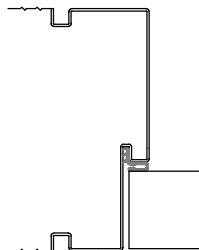
Variante/Beispiel: Verbr./Schatten-Nut
