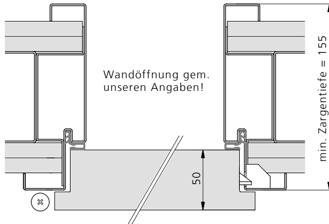
Variante/Beispiel: Spiegelverbreiterung
