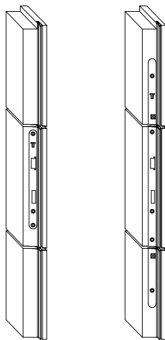
Einsteckschloss, 4-Punkt-Verriegelung
