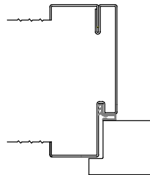
Variante/Beispiel: Stoss im Spiegel
