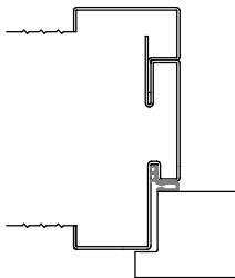
Variante/Beispiel: Stoss in der Leibung
