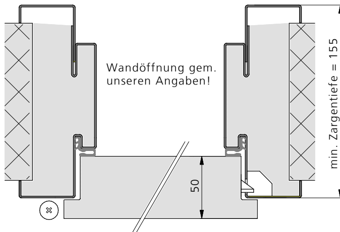
Variante/Beispiel: Stoss in der Leibung
