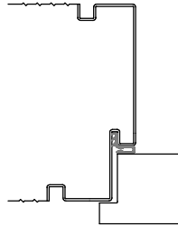
Variante/Beispiel: Schatten-Nut
