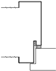
Variante/Beispiel: Spiegelverbreiterung
