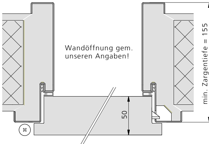
Variante/Beispiel: Spiegelverbreiterung
