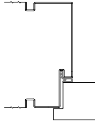
Variante/Beispiel: Verbr./Schatten-Nut
