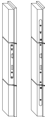
Einsteckschloss, 4-Punkt-Verriegelung
