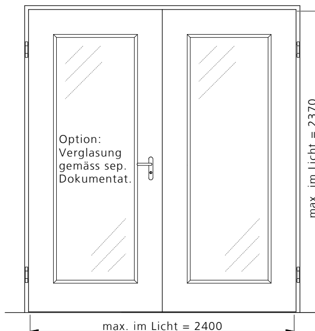
Variante/Beispiel: Verbr./Schatten-Nut
