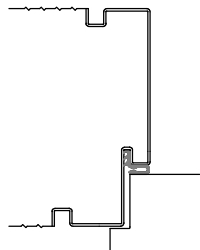
Variante/Beispiel: Schatten-Nut
