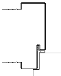
Variante/Beispiel: Spiegelverbreiterung
