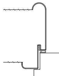
Variante/Beispiel: Rundspiegel
