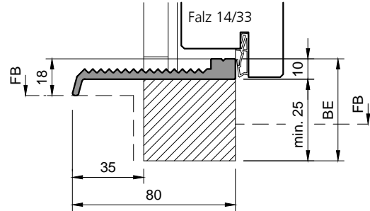
Typ: GS-TT (für Aussentüren)
