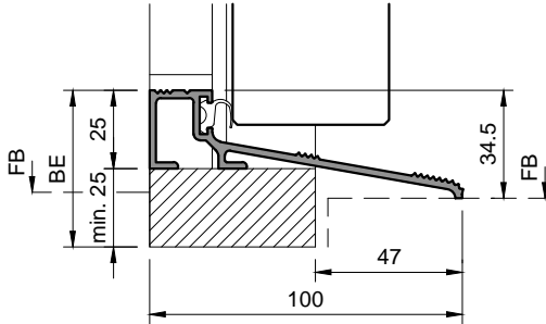
Typ: GS-165 (für Aussentüren, gegenöffnend) Achtung: Rahmendicke fix 53mm!
