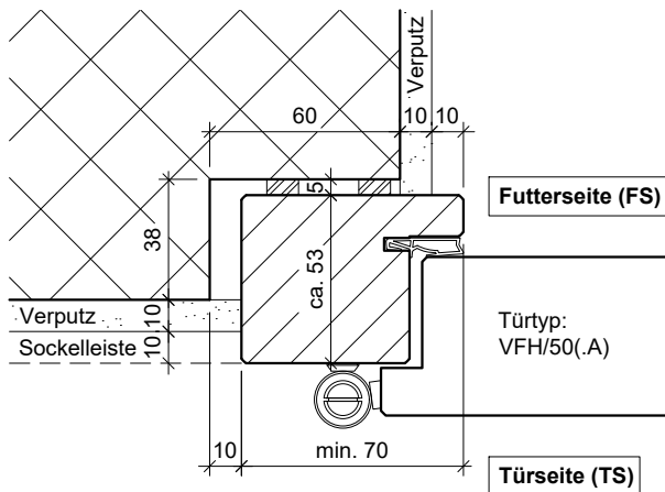
Typ RD17-40, Variante 3 Futter- und Türseite verputzt
