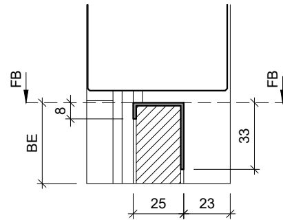
Typ: V-SP25 (Edelstahl Abdeckprofil)
