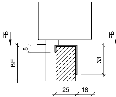
Typ: V-SP25 (Edelstahl Abdeckprofil)
