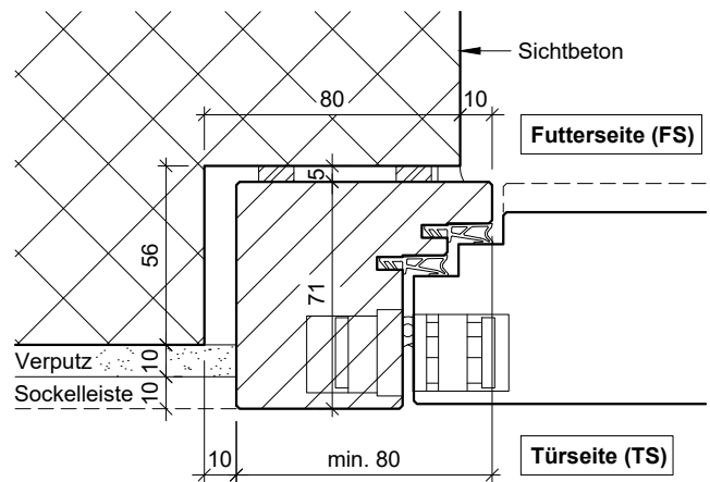
RDDS14-48/10 Variante 2 Futterseite Sichtbeton, Türseite verputzt
