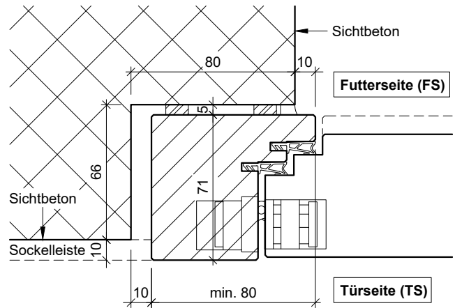
RDDS14-48/10 Variante 1 Futter- und Türseite Sichtbeton
