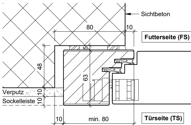
RDDS14-43/10 Variante 2 Futterseite Sichtbeton, Türseite verputzt
