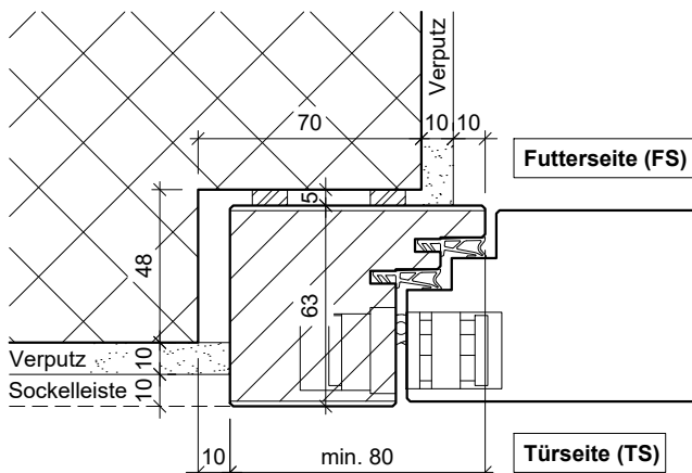
RDDS14-43/10 Variante 3 Futter- und Türseite verputzt
