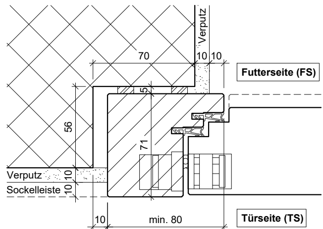
RDDS14-48/10 Variante 3 Futter- und Türseite verputzt
