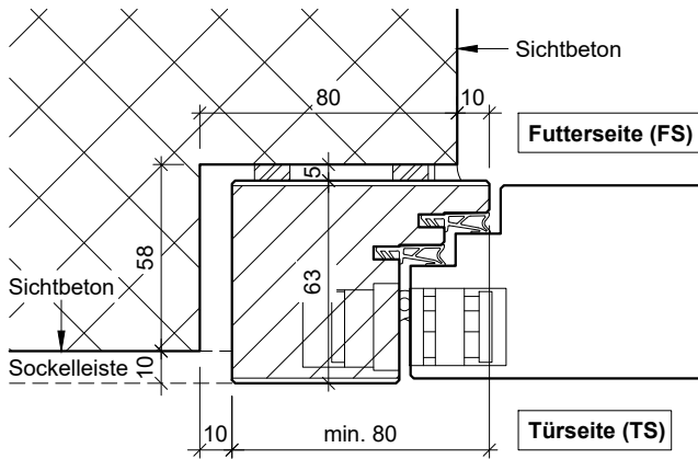
RDDS14-43/10 Variante 1 Futter- und Türseite Sichtbeton
