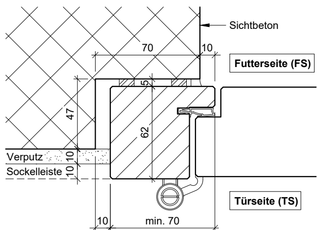
RDS17-48 Variante 2 Futterseite Sichtbeton, Türseite verputzt
