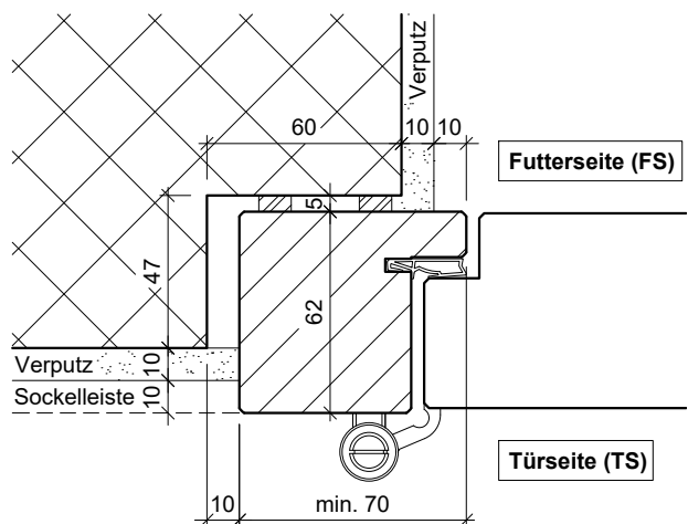
RDS17-48 Variante 3 Futter- und Türseite verputzt
