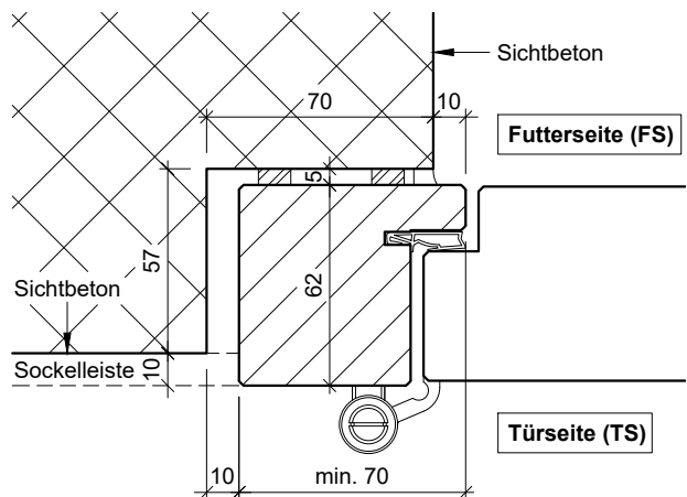
RDS17-48 Variante 1 Futter- und Türseite Sichtbeton
