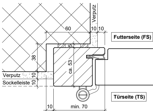
RDS17-43 Variante 3 Futter- und Türseite verputzt
