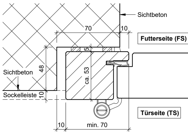
RDS17-43 Variante 1 Futter- und Türseite Sichtbeton
