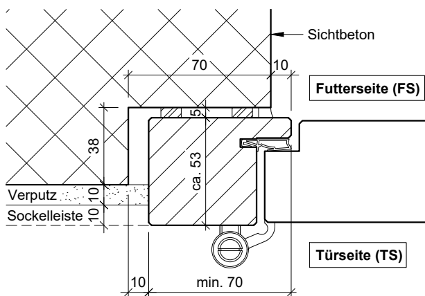
RDS17-43 Variante 2 Futterseite Sichtbeton, Türseite verputzt
