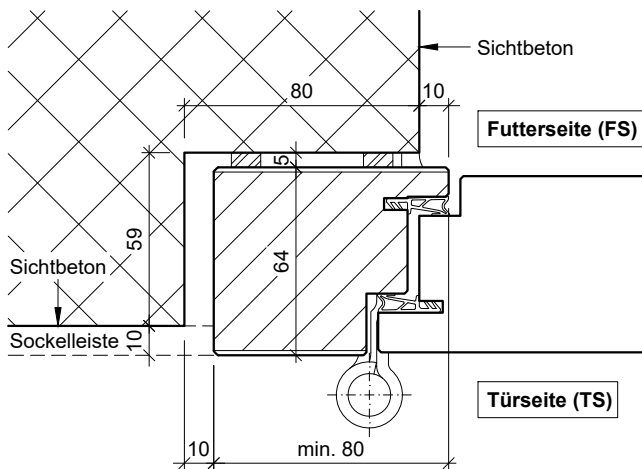
RDS14-21/33 Variante 1 Futter- und Türseite Sichtbeton
