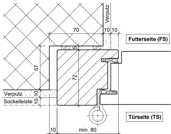
RDS14-21/40 Variante 3 Futter- und Türseite verputzt
