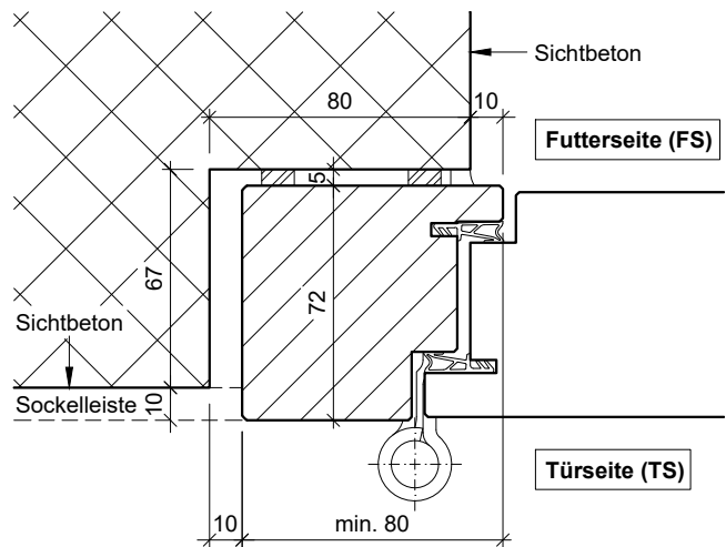
RDS14-21/40 Variante 2 Futterseite Sichtbeton, Türseite verputzt
