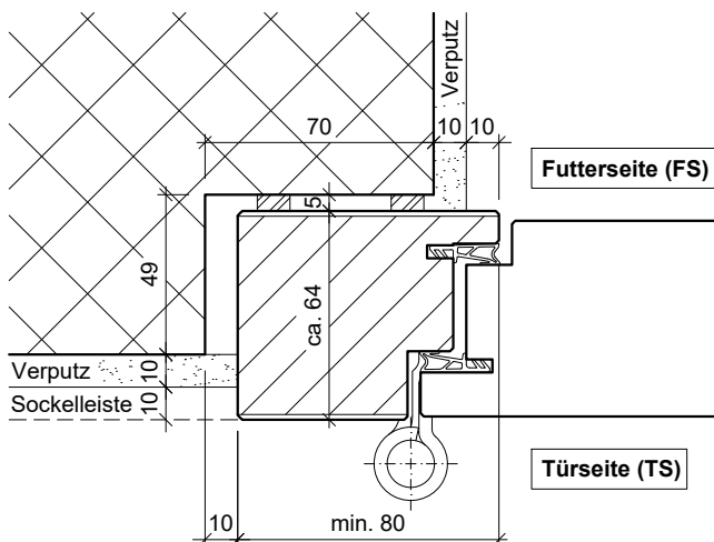
RDS14-21/33 Variante 3 Futter- und Türseite verputzt
