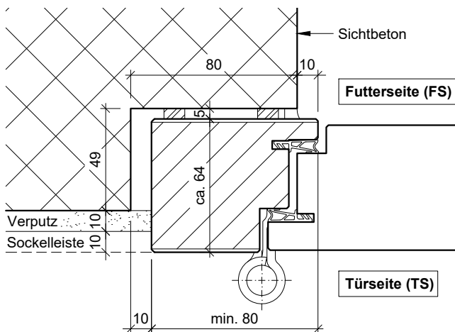
RDS14-21/33 Variante 2 Futterseite Sichtbeton, Türseite verputzt
