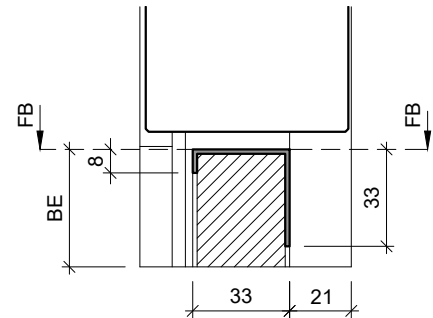
Typ: V-SP33 (Edelstahl Abdeckprofil)
