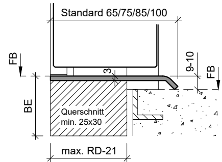
Typ: KSR.B (Alu Konter-Umbauschwelle)
