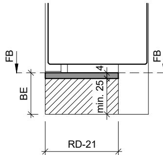
Typ: KSA.B (Alu Konter-Schwelle) Schwellenbreite = Holzdicke
