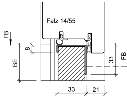
Typ: SP33 (Edelstahl Abdeckprofil)
