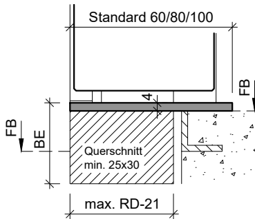
Typ: KSA.B (Alu Konter-Umbauschwelle)
