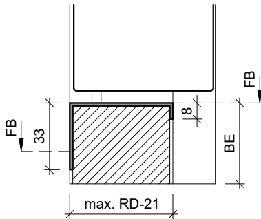
Typ: KSP.B (Sonderanfertigung) (Edelstahl Konter-Abdeckprofil)
