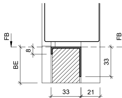
Typ: V-SP33 (Edelstahl Abdeckprofil)
