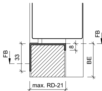
Typ: KSP.B (Sonderanfertigung) (Edelstahl Konter-Abdeckprofil)
