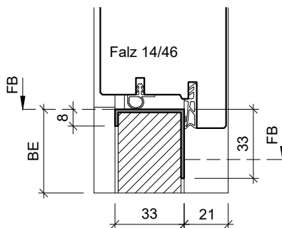
Typ: SP33 (Edelstahl Abdeckprofil)
