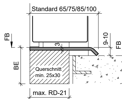
Typ: KSR.B (Alu Konter-Umbauschwelle)
