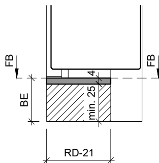
Typ: KSA.B (Alu Konter-Schwelle) Schwellenbreite = Holzdicke
